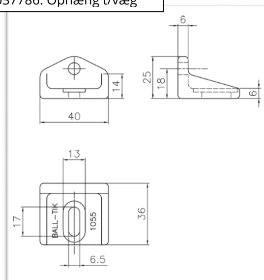
9037786: Ophæng t/væg
