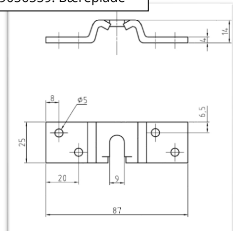
9056559: Bæreplade
