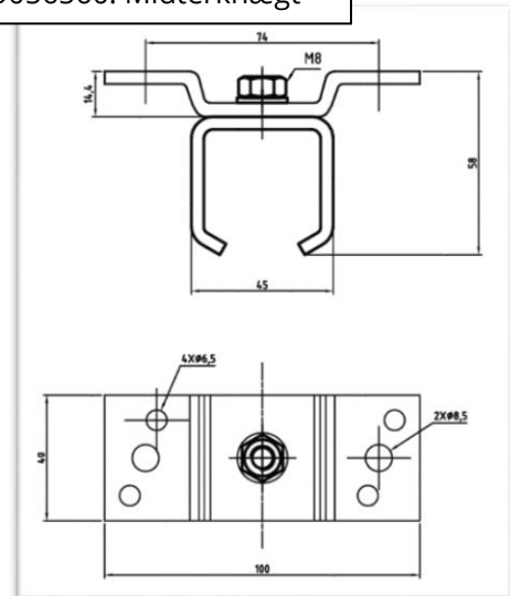
9056560: Midterknægt
