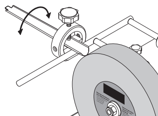
Vorrichtung für Röhren und Hohleisen (mit 100) 55, Bestell-Nr. 8949 0706
