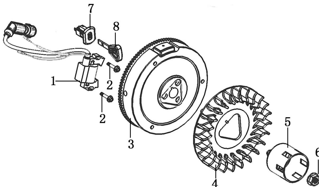
FIG. 7 Tænding
