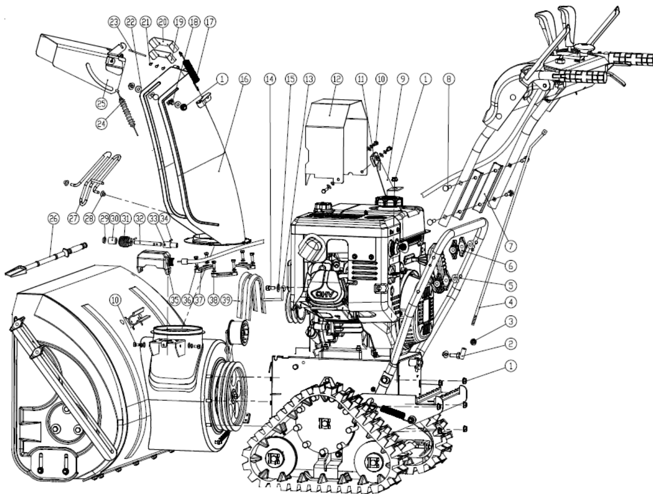
Fig 1 Hovedmaskine
