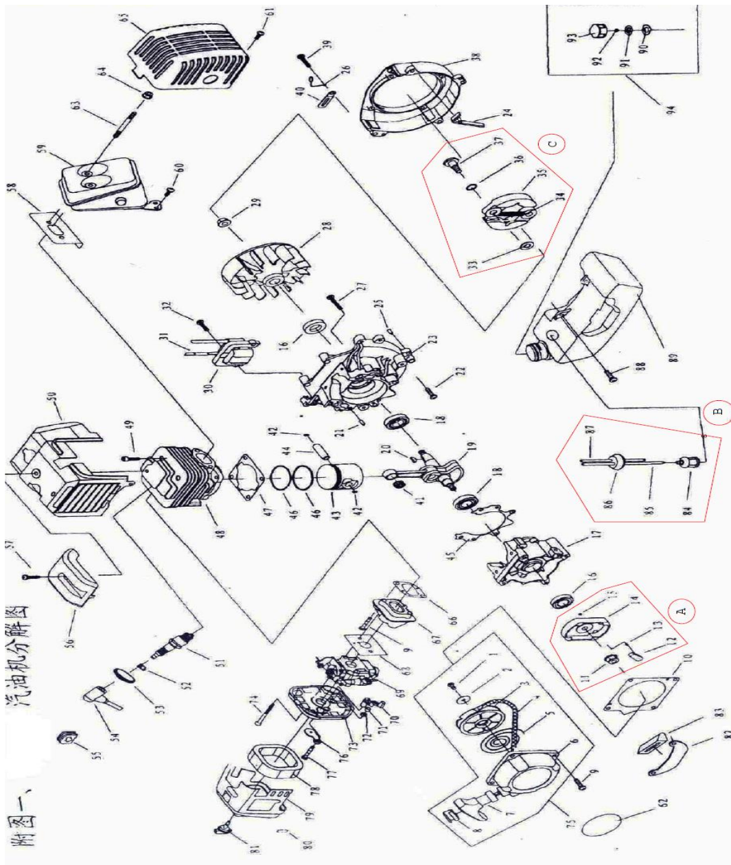
Fig. 1/Pælebor motor
