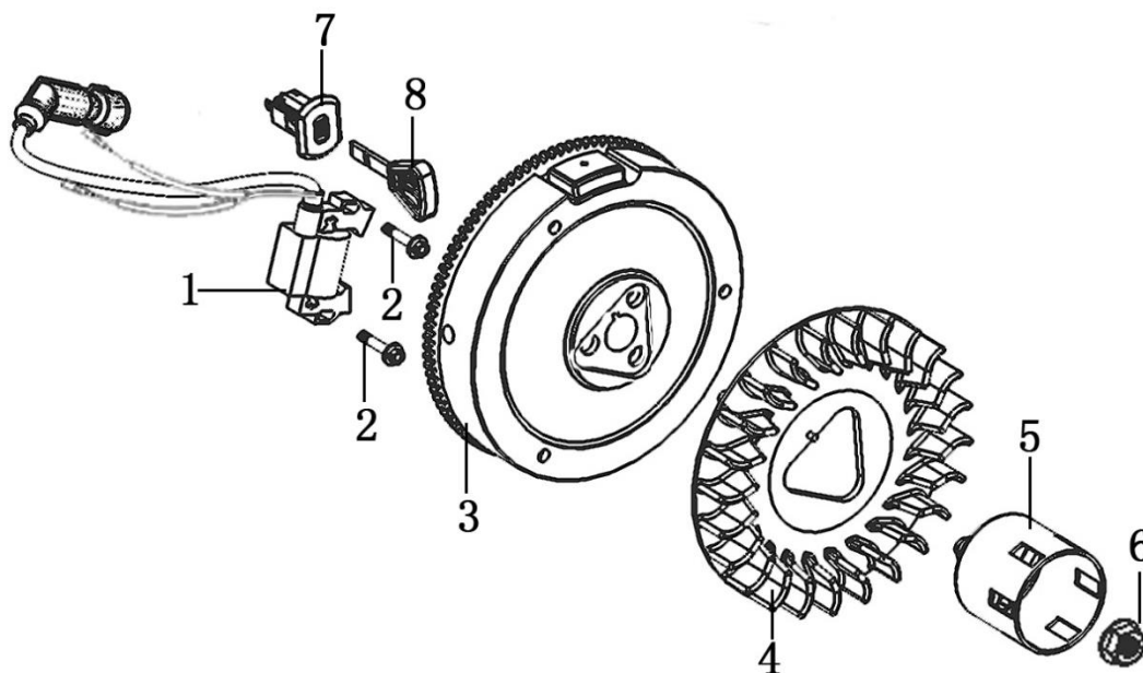
FIG. 7 Tænding
