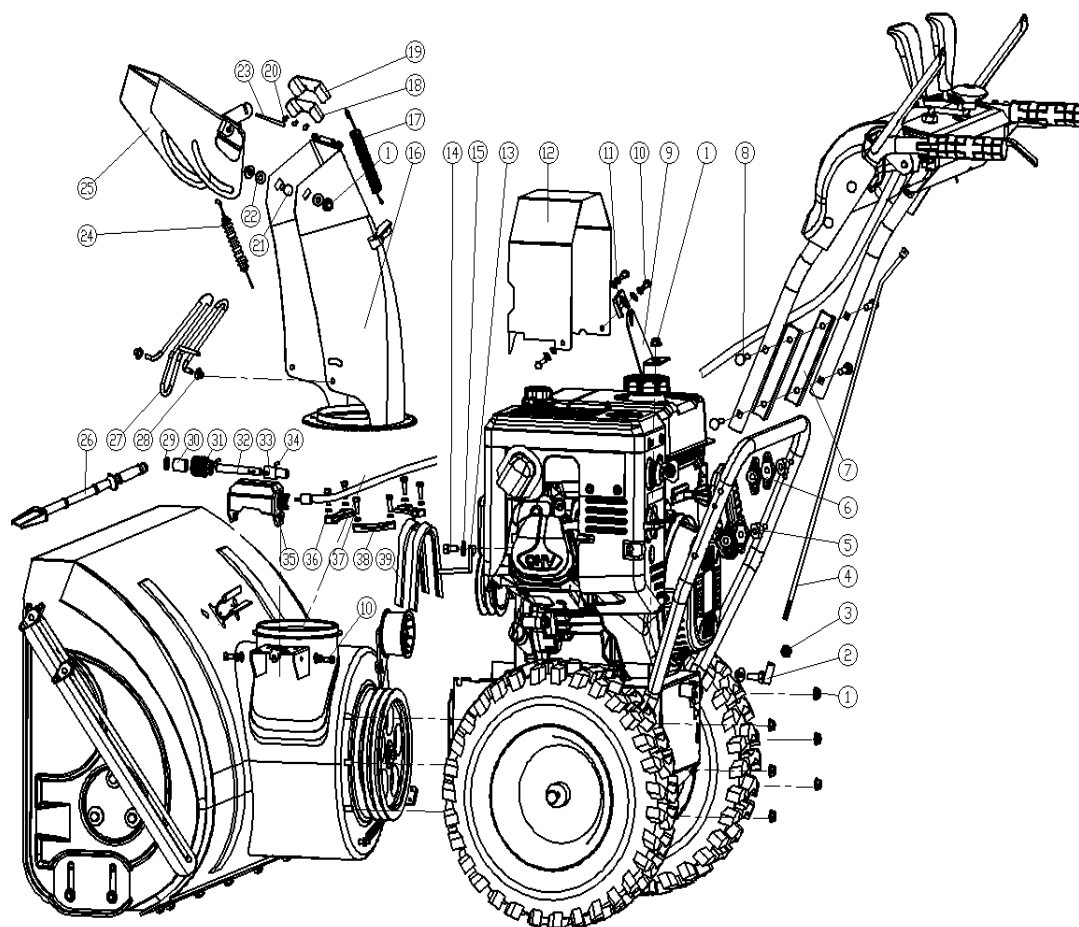
Fig 1 Hovedmaskine
