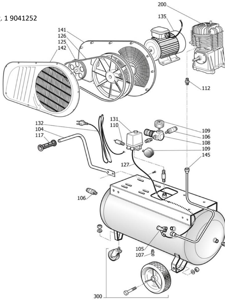
Fig. 2 Kompressorblok
