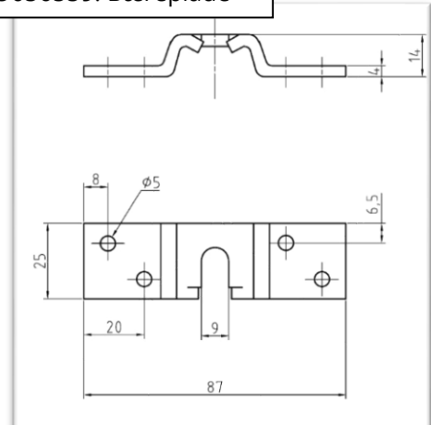
9056559: Bæreplade
