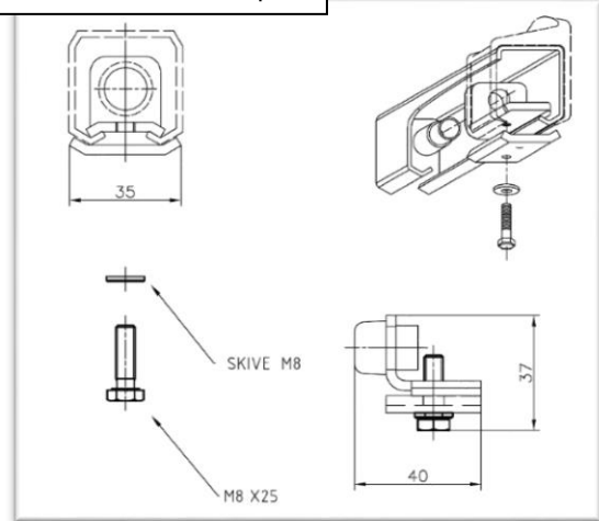
9056560: Midterknægt
