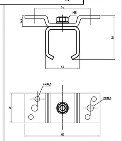
9056560: Midterknægt
